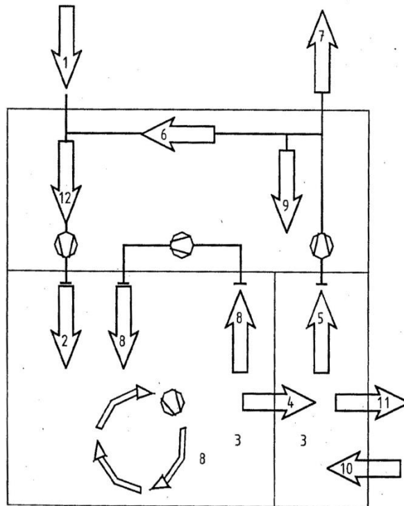
Figuur 1 - Illustratie van de luchttypen volgens NEN 13779: 2004.
